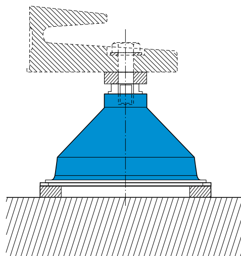
Installation avec rondelles
