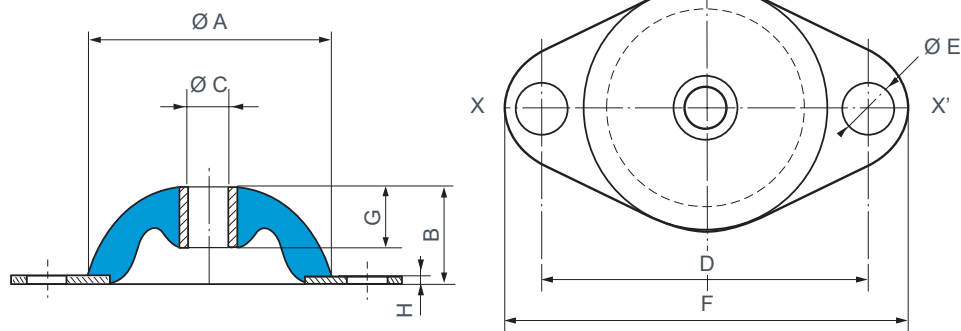
Coupe XX'
