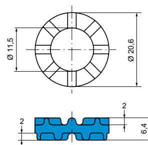
Rondelles
